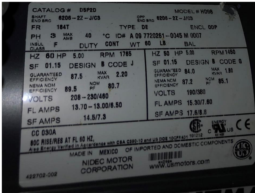
AHU-6
